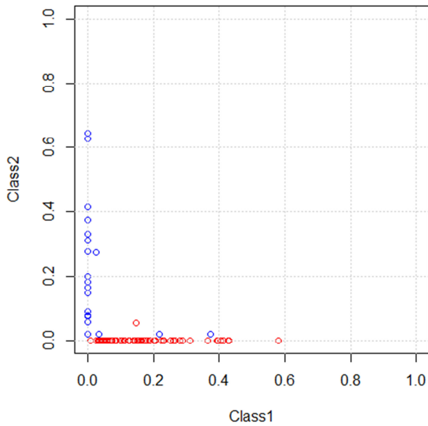
DD-Plot (zonoid): ecoli_cpvspp
