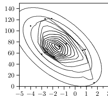
(d) zonoid-Mahalanobis depth with \beta = 0.33
